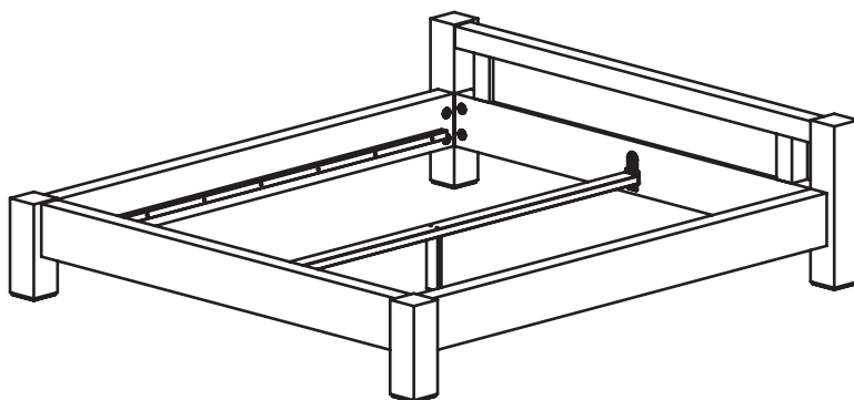
TYP 98/2000 - S 2240/W 610/G 2244 TYP 98/1800 - S 2040/W 610/G 2244 TYP 98/1600 - S 1840/W 610/G 2244 TYP 98/1400 - S 1640/W 610/G 2244
