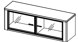
Typ 14 B/H/T 1235/408/350 106401424
